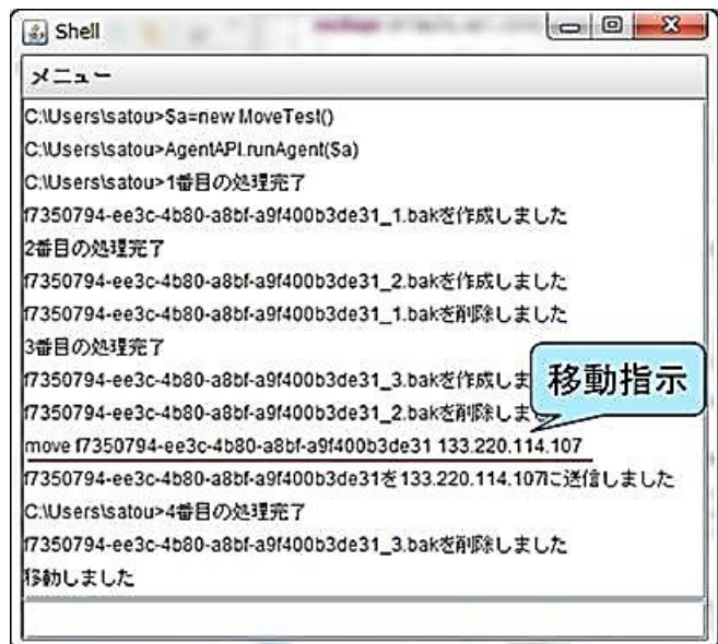
図 6. 送信側マシンの実行結果
