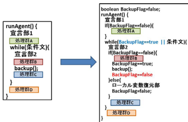
図 4.ループ文の中に backup メソッドがある場合の変換
