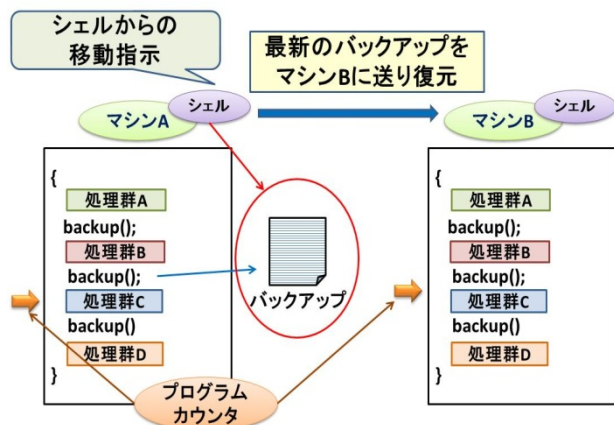
図 1. バックアップを利用したエージェント移動
