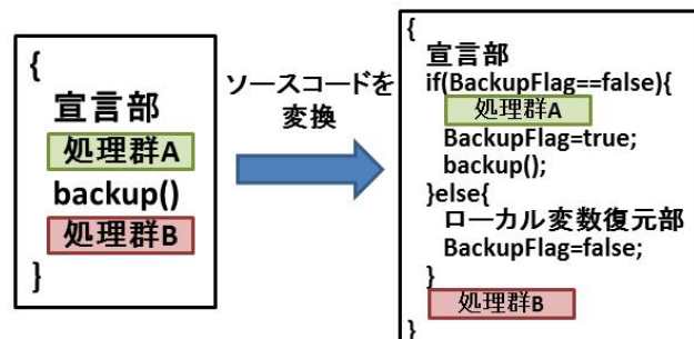
図 2. バックアップを含むソースコードの変換
