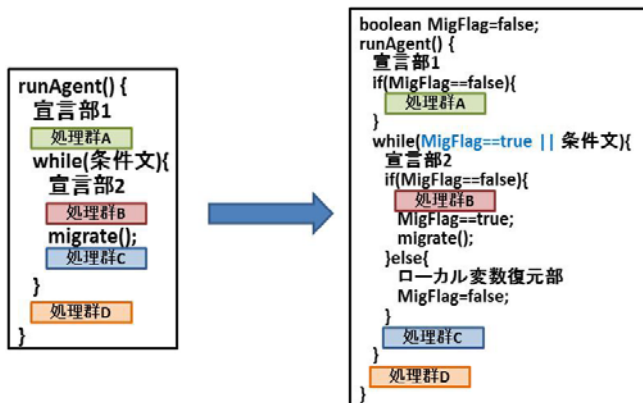
図 3.ループ文の中に migrate メソッドがある場合の変換
