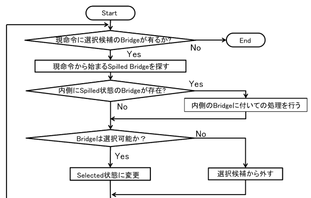
図3 Bridge Select のフローチャート
