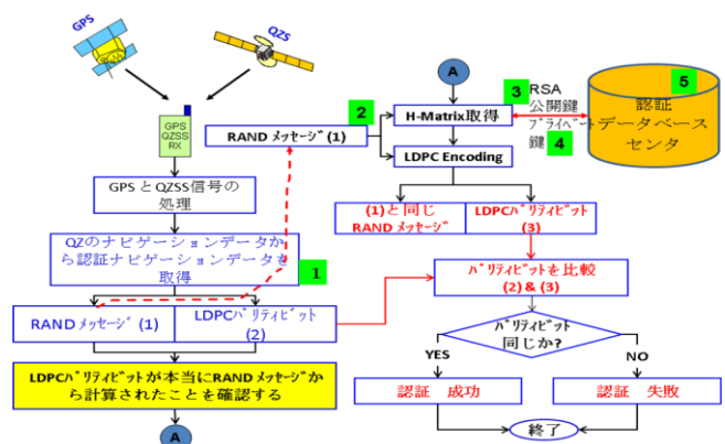
図7 受信機での信号認証手順の詳細
