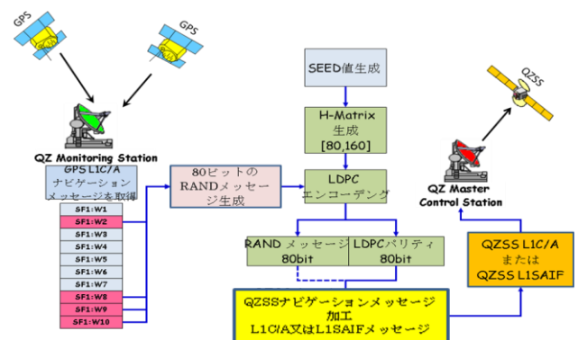
図3 信号送信における認証メッセージの概念
