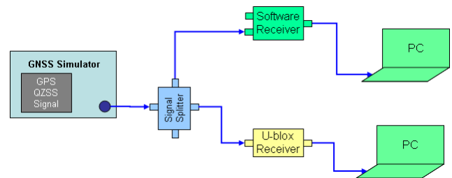
図 11 GNSS 信号シミュレータと u-blox 受信機とソフトウェア受信機を利用した認証シミュレーション実験例
