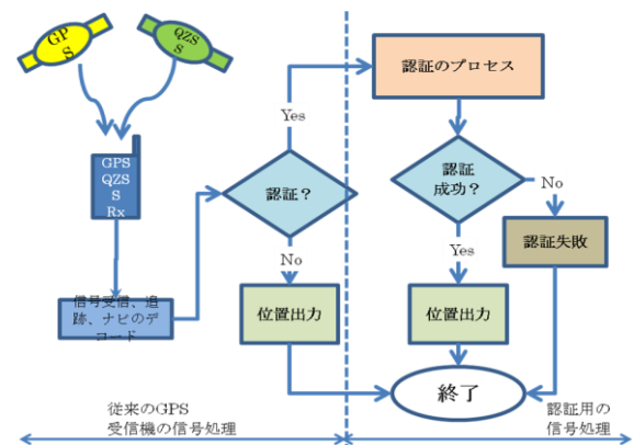
図6 受信機での信号認証の概念
