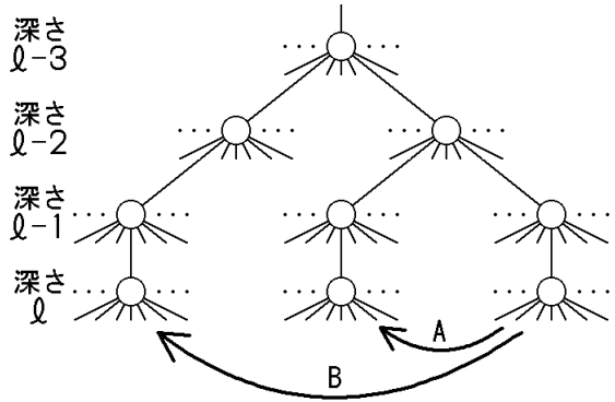
図 3. 共有する祖先と同一局面間の距離の関係
