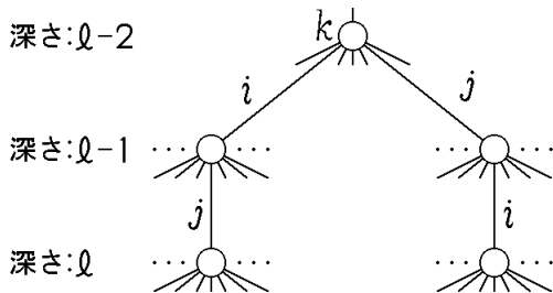
図 2. 2 世代前の祖先を共有する同一局面の例
