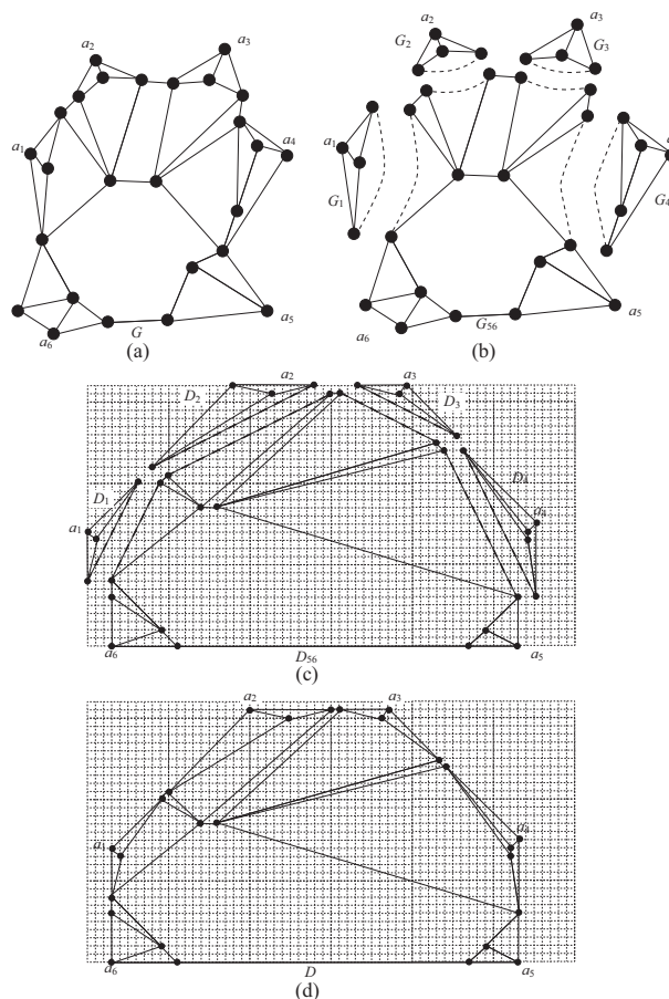
図 1: (a) 平面グラフ G , (b) グラフ G_1, G_2, G_3, G_4 および G_{56} , (c) 描画 D_1, D_2, D_3, D_4 および D_{56} , (d) G の描画 D 。
