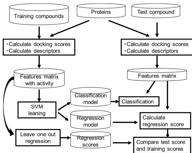
図 2. 機械学習の流れ
