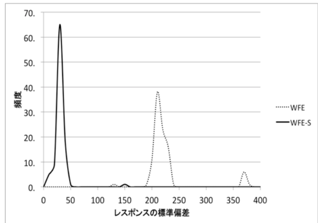
図 9: レスポンスの標準偏差の分布
