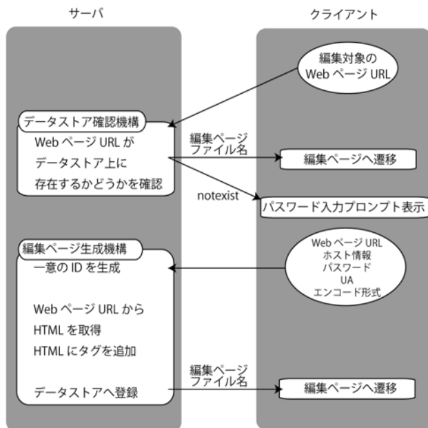
図 7: ブックマークレットの動作詳細
