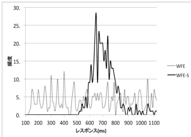
図 8: レスポンスの分布
