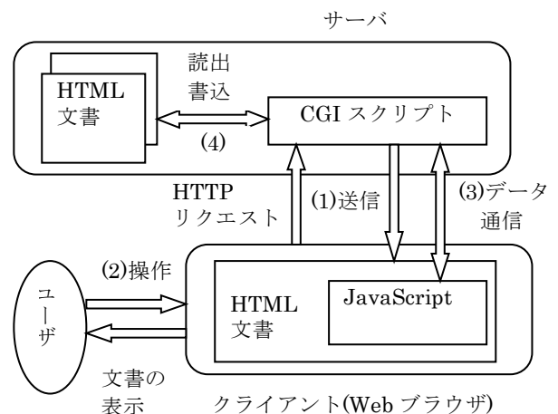
図 1. WFE システムの概観
