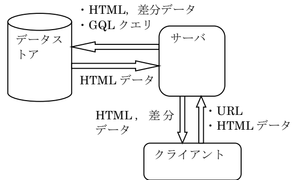
図 6. データストアを用いた HTML データの保管
