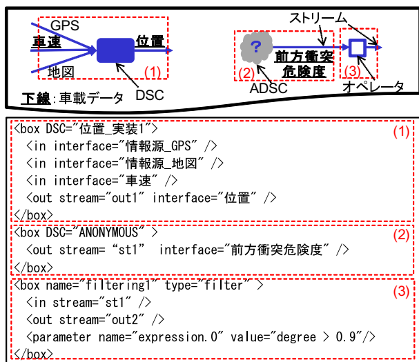
図 4: ユーザによるクエリの記述
