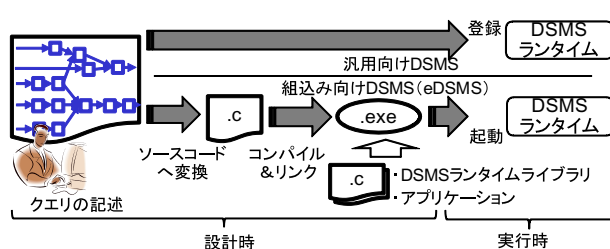
図 2: 汎用向け DSMS と eDSMS との違い
