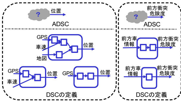
図 3: DSC の定義とそのグルーピング, ADSC
