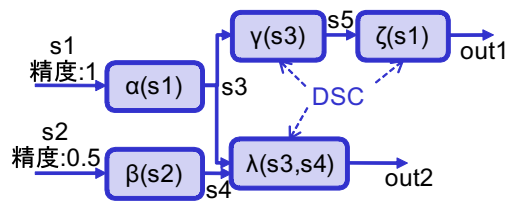
図 6: 精度の見積もり
