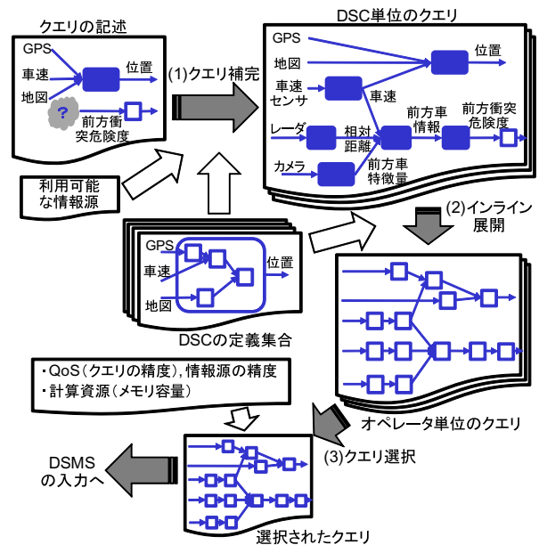
図 5: 提案手法の処理の流れ
