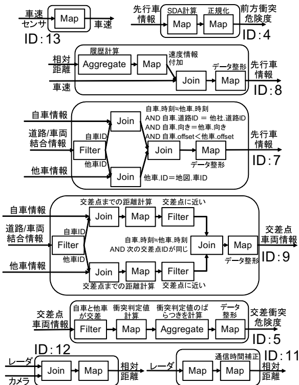
図 7: DSC の定義の例
