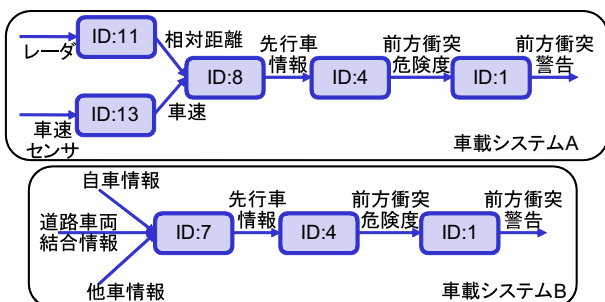
図 8: 構築された DSC 単位のクエリ
