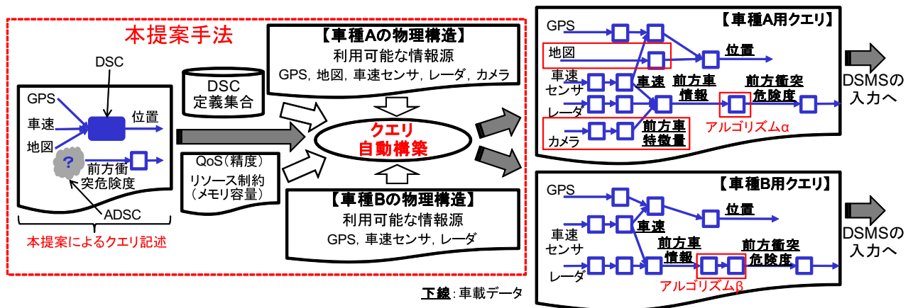
図 1: 提案手法によるクエリ記述
