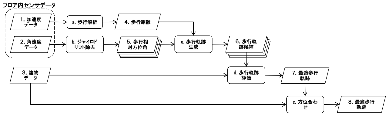
図 3. 歩行の始点終点座標が同一の場合の推定方式
