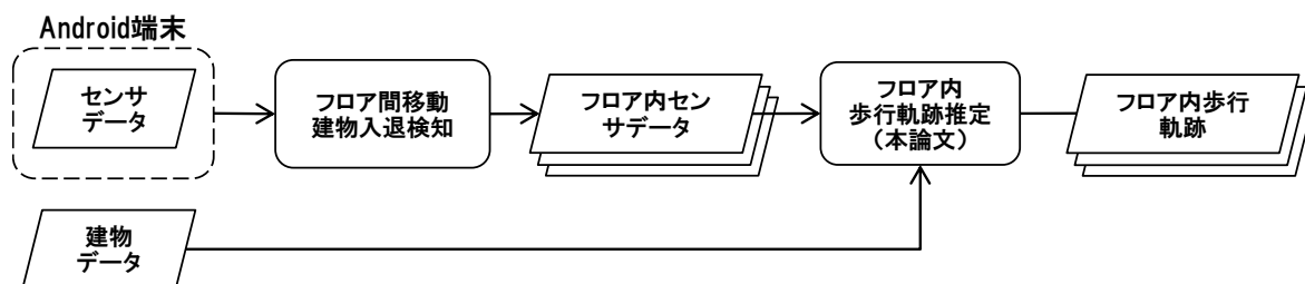
図 2. 屋内歩行軌跡推定方式の構成
