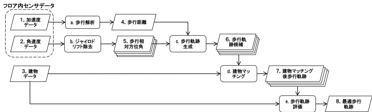
図 4. 歩行の始点終点座標が異なる場合の推定方式
