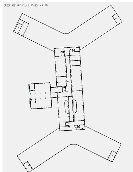
図6 歩行環境の外形図 (中央の長方形が5階フロア, 20m×60m)
