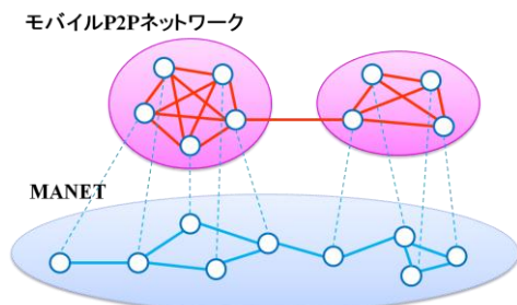
図 3 分散ネットワーク型リソース管理手法
