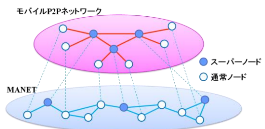
図 2 スーパーノード型リソース管理手法
