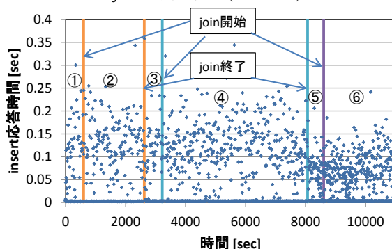
図8 書き込み性能と各ノードのjoin時間の関係(4台並列)
