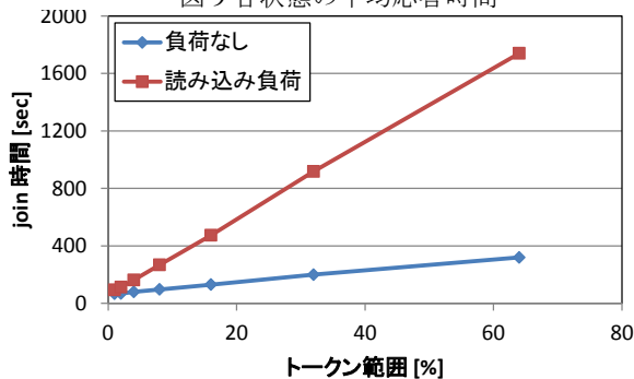
図10 トークン範囲とjoin時間の関係
