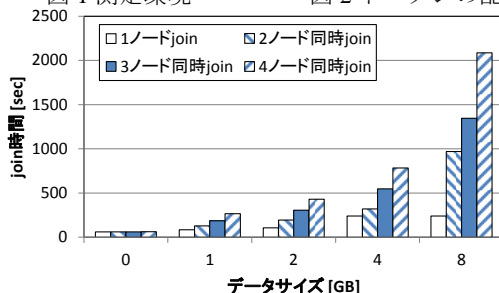
図3 データサイズと各ノードのjoin時間の関係(複数台並列)
