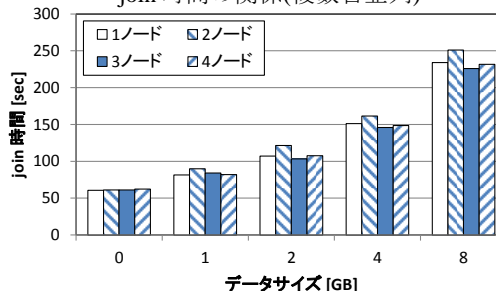
図4 データサイズと各ノードのjoin時間の関係(順次)
