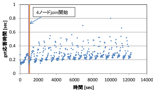
図7 読み込み性能と各ノードのjoin時間の関係(4台並列)
