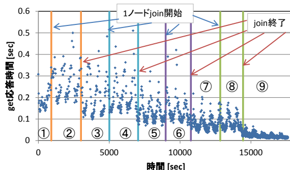
図5 読み込み性能と各ノードのjoin時間の関係(順次)
