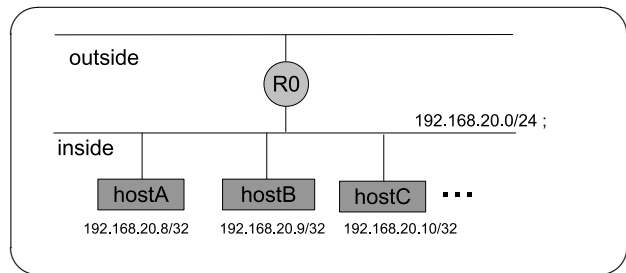
図 2: 論理ネットワーク図の例
