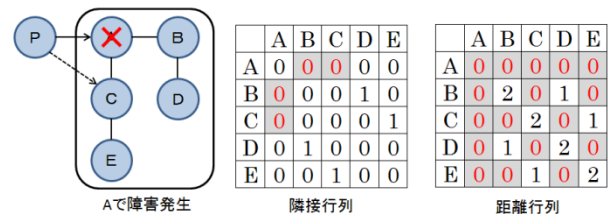
Fig. 4 要素 A で障害発生時の隣接行列と距離行列
