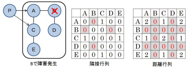
Fig. 3 要素 B で障害発生時の隣接行列と距離行列
