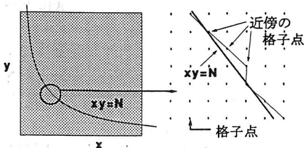
図 1 双曲線の近傍の格子点
