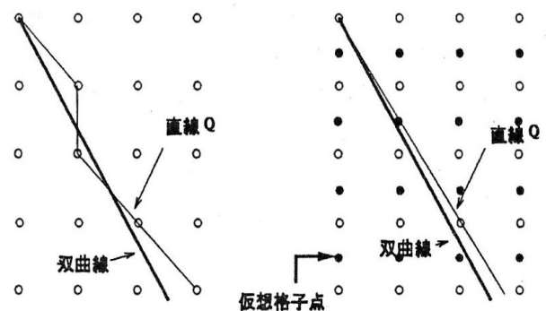
図 2 仮想格子点の考慮
