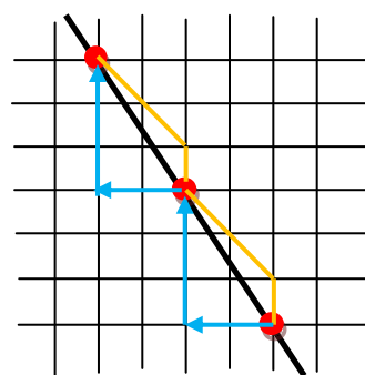
図 4 図 3 における P の拡大図
