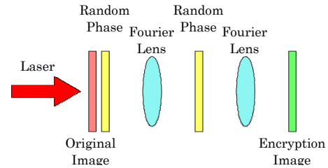
図 5 二重ランダム位相暗号化法
