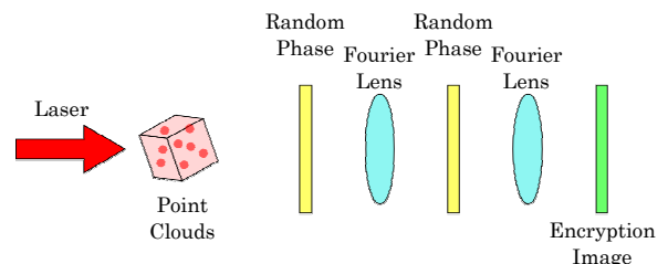
図 6 新しい光暗号化法
