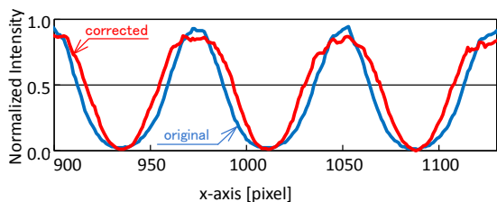
図 3 補正前後の正弦波比較
