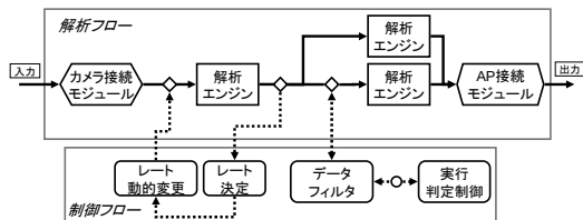
図 2 解析・制御フロー例
