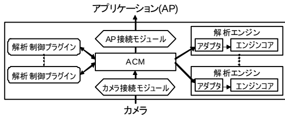
図 1 ACM アーキテクチャ概要図
