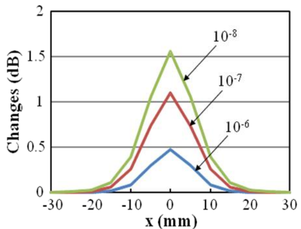
図 2 (b) \mu_a 変化と受信信号強度変化 (CSF 有、 \rho = 2\text{mm} )
