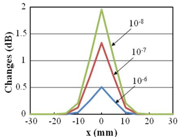
図 2 (a) \mu_a 変化と受信信号強度変化 (CSF 無し、 \rho = 2\text{mm} )
