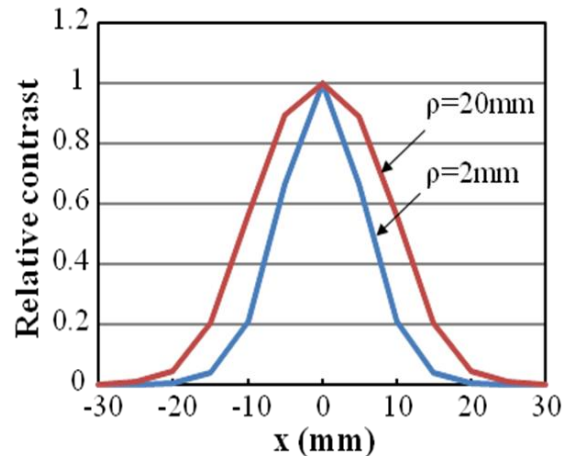
図 3 (b) 光源・検出器間隔とコントラスト(CSF 有)
