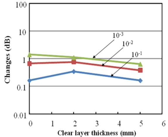
図 4 (b) \rho=20\text{mm} の最大感度の CSF 厚み依存性
