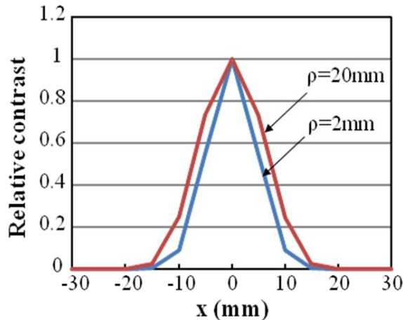
図 3 (a) 光源・検出器間隔とコントラスト(CSF 無)
