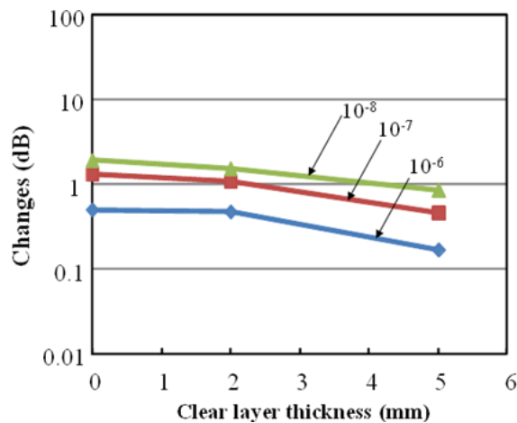
図 4 (a) \rho=2\text{mm} の最大感度の CSF 厚み依存性
