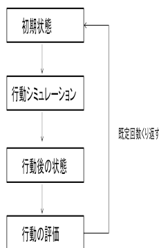
図 4: モンテカルロ法のアルゴリズム
