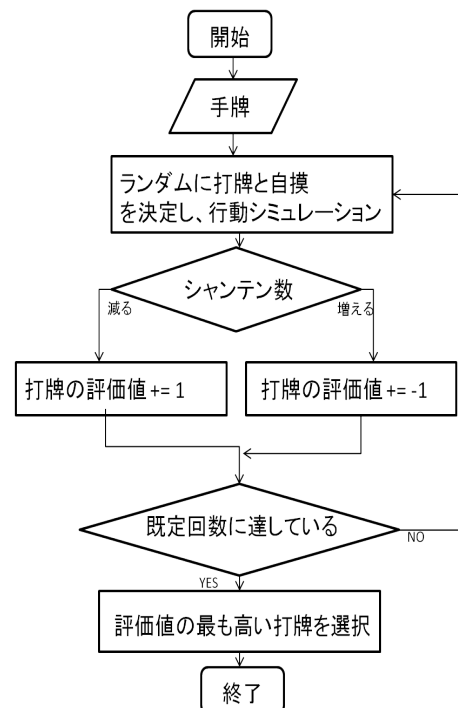
図 5: 評価値増減法フローチャート
