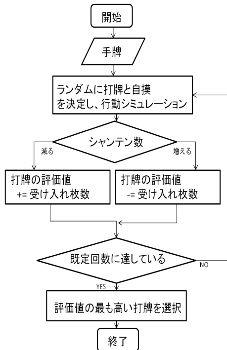
図 6: 評価値増減法フローチャート
