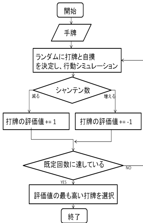
図 1: 遺伝的アルゴリズムのフローチャート
