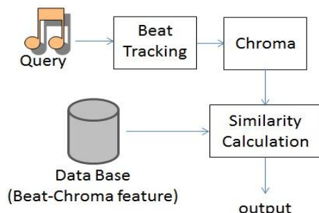
図 1: Ellis 手法[5]の処理の流れ
