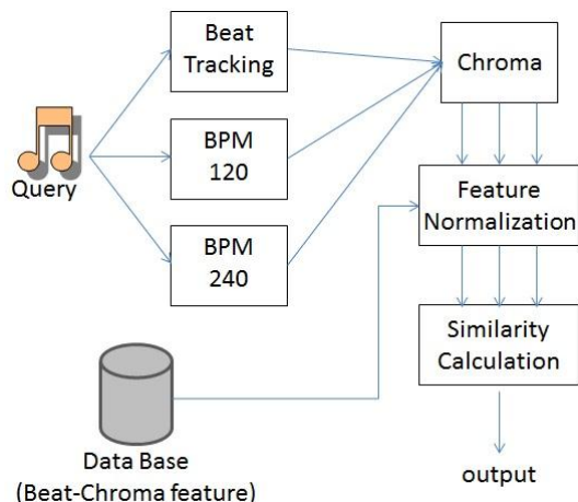
図 3: 提案手法の処理の流れ
