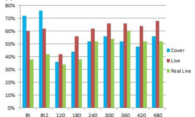
図 2: 各ビート情報取得手法による楽曲同定精度の変化
