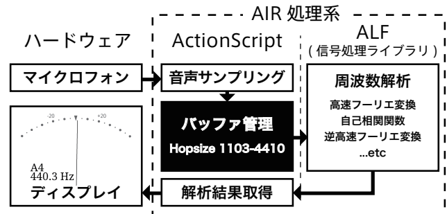
図 1 チューナアプリケーションの構成
