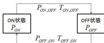
図 1 2 状態遷移における動的電源制御例 [1]
