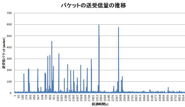
図 2 パケット送受信量の推移
