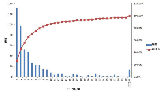
図 3 得られたデータを自身の IP アドレスかつポート番号が 80 でフィルタリングし、データリクエスト間隔の累積確率を、リクエスト間隔ごとにプロットした。
