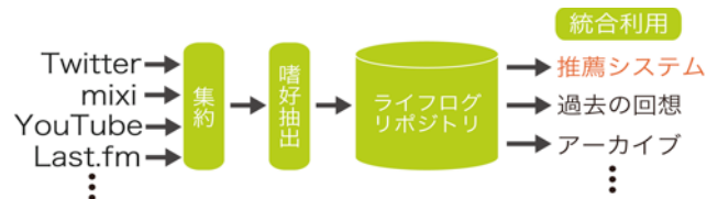
図2 ライフログリポジトリ
