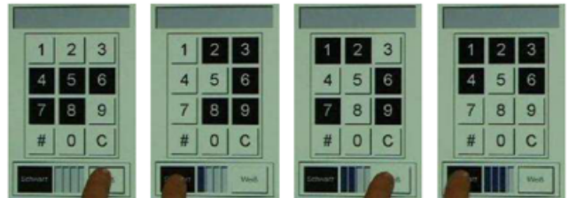
図4 Roth氏らによる PIN-ENTRY METHOD
