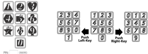
図3 高田氏による fakePointer
