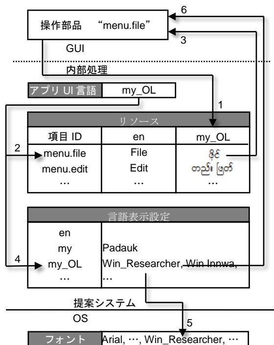
図 4 提案システムにおけるビルマ語 UI 処理
