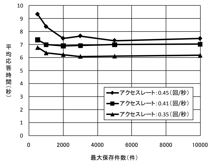
図5 最大保存件数による平均応答時間の変化
