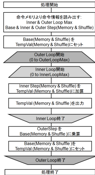
図2 2-D GAGの制御方法
