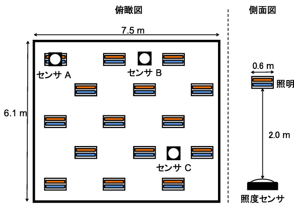
図 3: 実験環境
