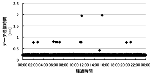
図 2: 通信時間 (6/7 火)
