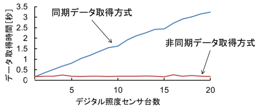
図3 デジタル照度センサのデータ取得時間
