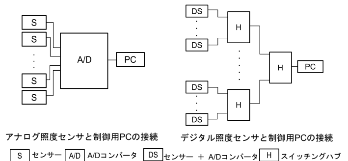
図2 接続方式の比較
