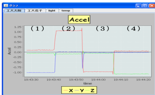
図 3: 3-axis Acceleration グラフ
