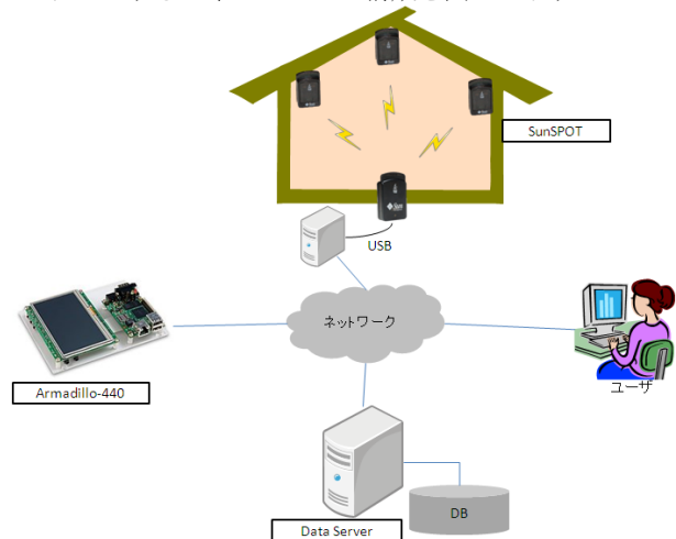
図2: システム構成の概要
