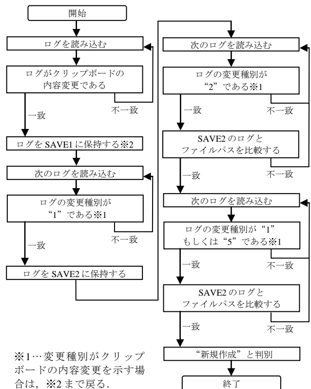
図 3 “新規作成” のログを対象とした解析手法の流れ
