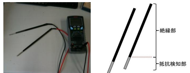
図2. 箸に DMM を装着した図、デバイス構成図
