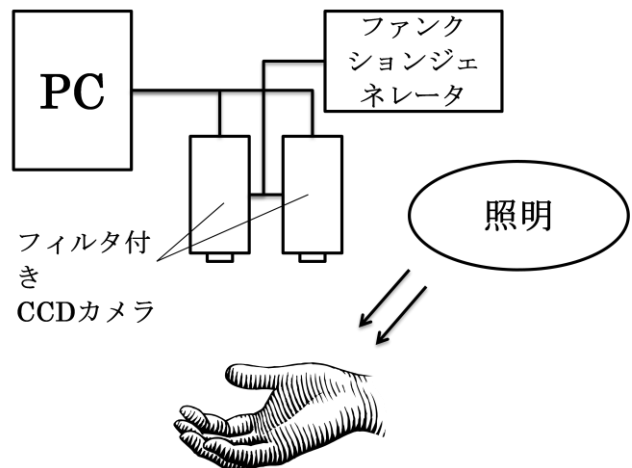
図1 従来の実験装置構成図
