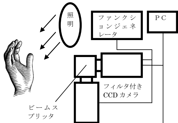
図2 本研究の実験方法
