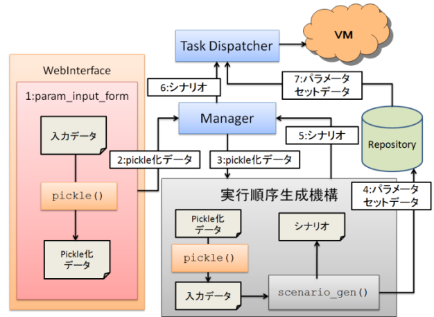
図4: 実行順序生成機構の構成
