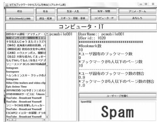
図 2. リアルタイムスパム判定システム
