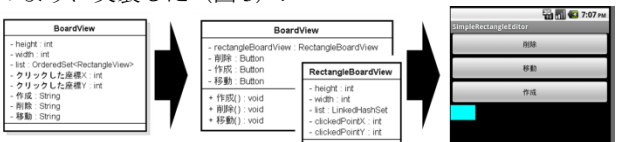
図5：出力構造をAndroidのUIと対応
