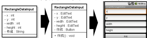
図4：入力構造をAndroidのUIと対応
