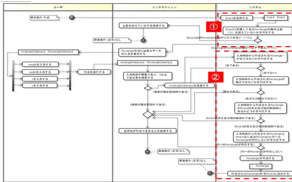
図1: 「長方形を作成する」サービスのアクティビティ図
