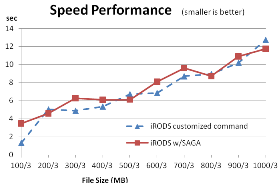
図 3. customized iget VS SAGA iRODS
