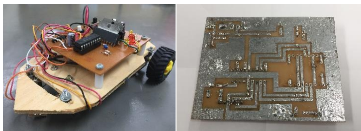
過去作製したラントレーサと基板
