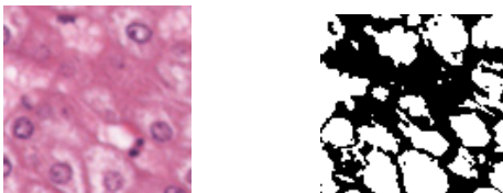
図 1 2 値化結果例
