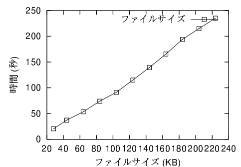
図8 計算時間
