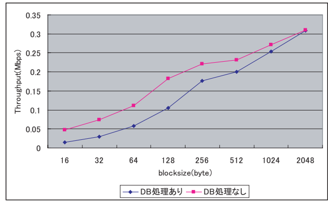
図 14 blocksize に対するスループット (DB 転送)
