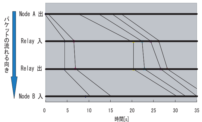
図 12 read/write なしの場合のパケットトレース
