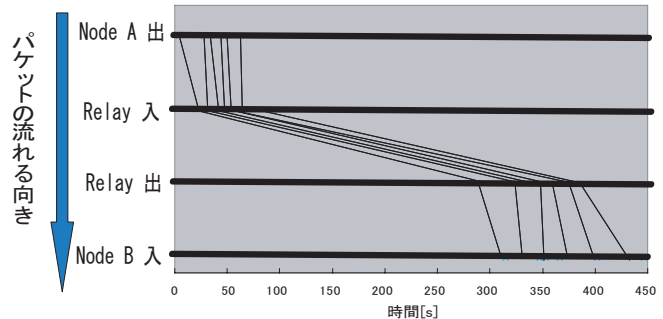
図 16 中継装置に DB 処理をさせた場合のパケットトレース
