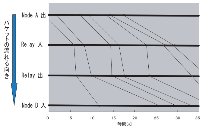
図 13 read/write ありの場合のパケットトレース
