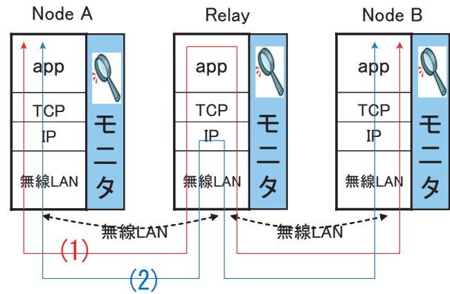
図 7 パケットの転送経路
