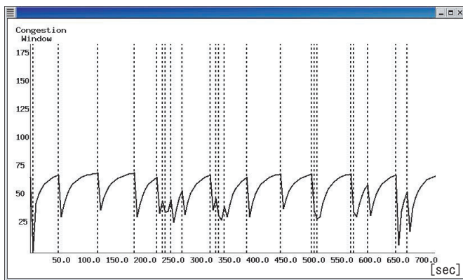
図 10 read/write ありの場合の輻輳ウィンドウ時間変化
