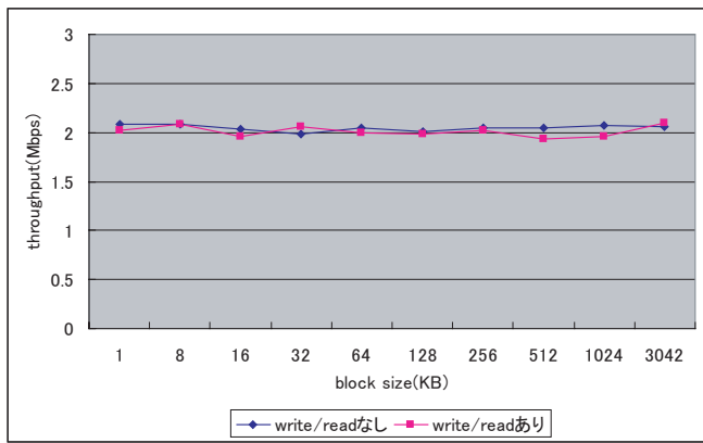
図 8 blocksize に対するスループット (read/write)
