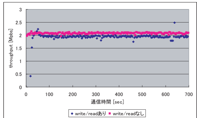
図 11 スループット時間変化
