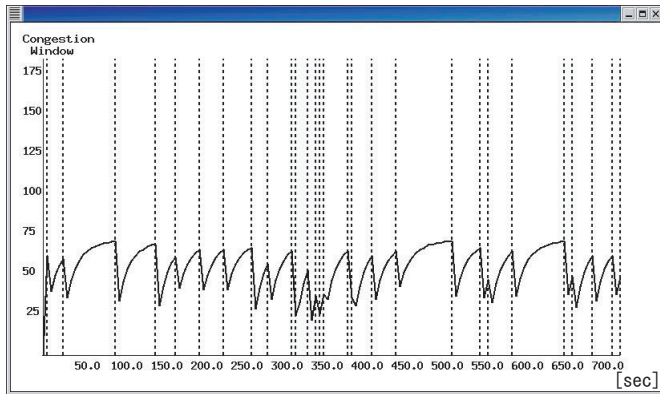
図 9 read/write なしの場合の輻輳ウィンドウ時間変化
