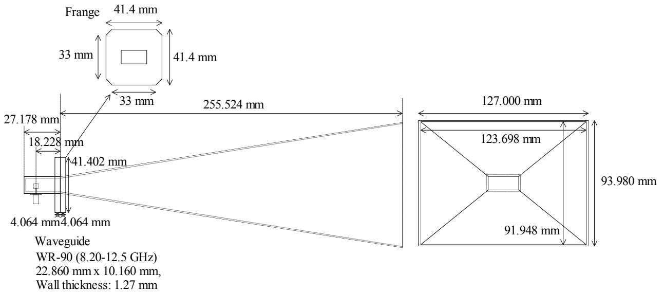
図 1 標準ホーンアンテナ(10 GHz, 20 dBi)
