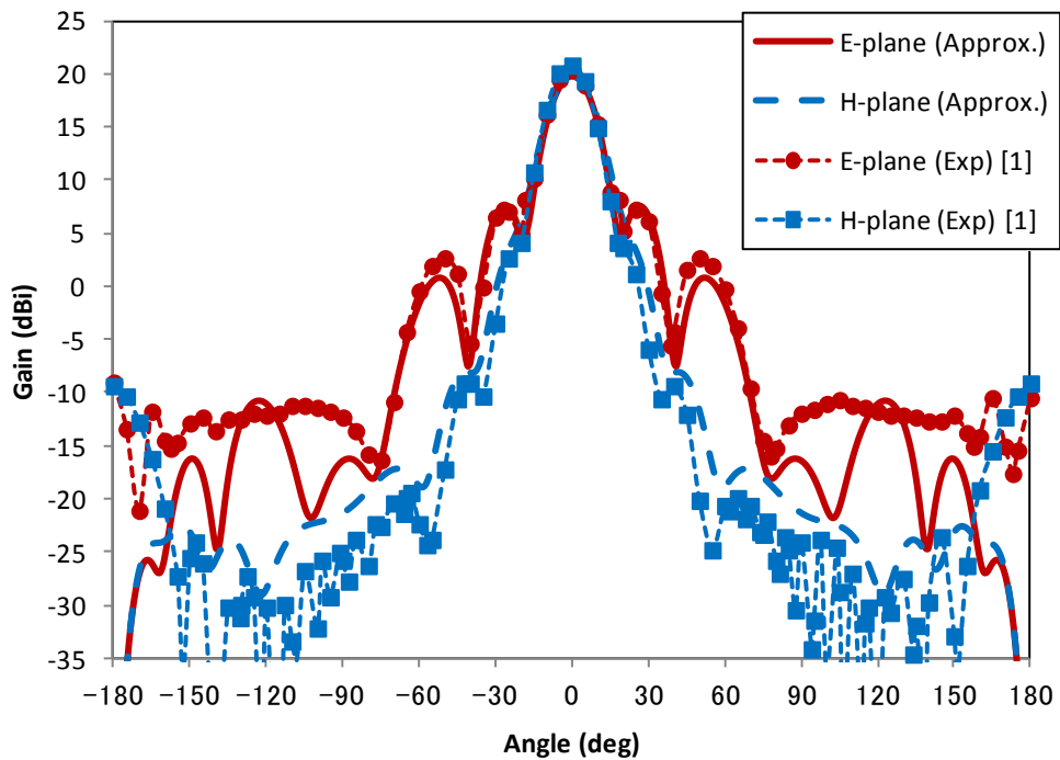
図 2 標準ホーンアンテナの利得指向性
