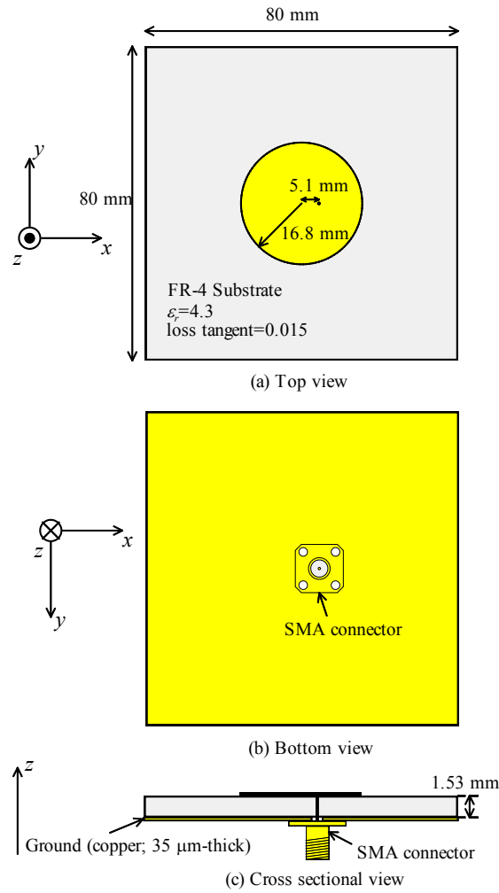
図 1 2.5GHz 帯 FR-4 基板円形パッチアンテナ
