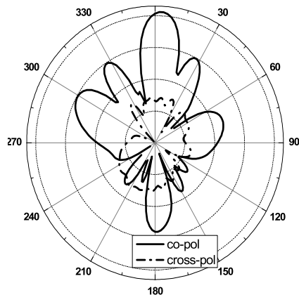
(b)H-plane
