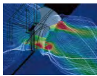
室外機搭載時のファンの風速解析結果
