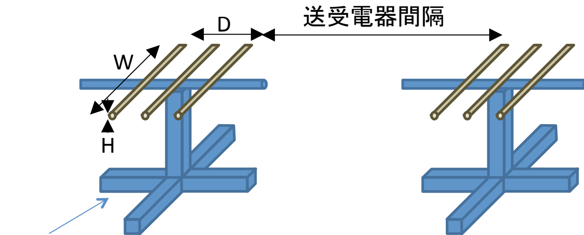
図3: 線状アンテナの例
