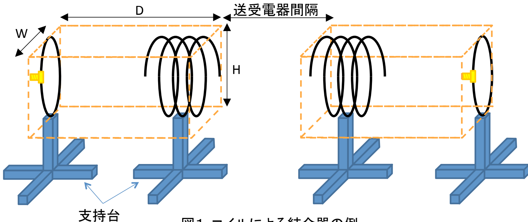
図1:コイルによる結合器の例
