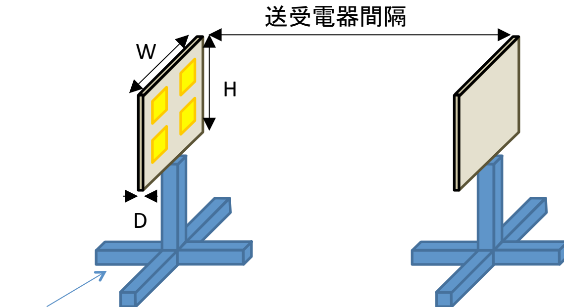
図2: 平面アンテナの例
