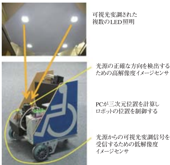
図7 可視光通信を用いたロボットの制御 (慶大, NEC)
